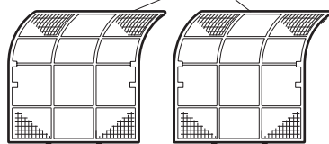
Фотокаталитический титан-апатитовый фильтр очистки воздуха (2)
