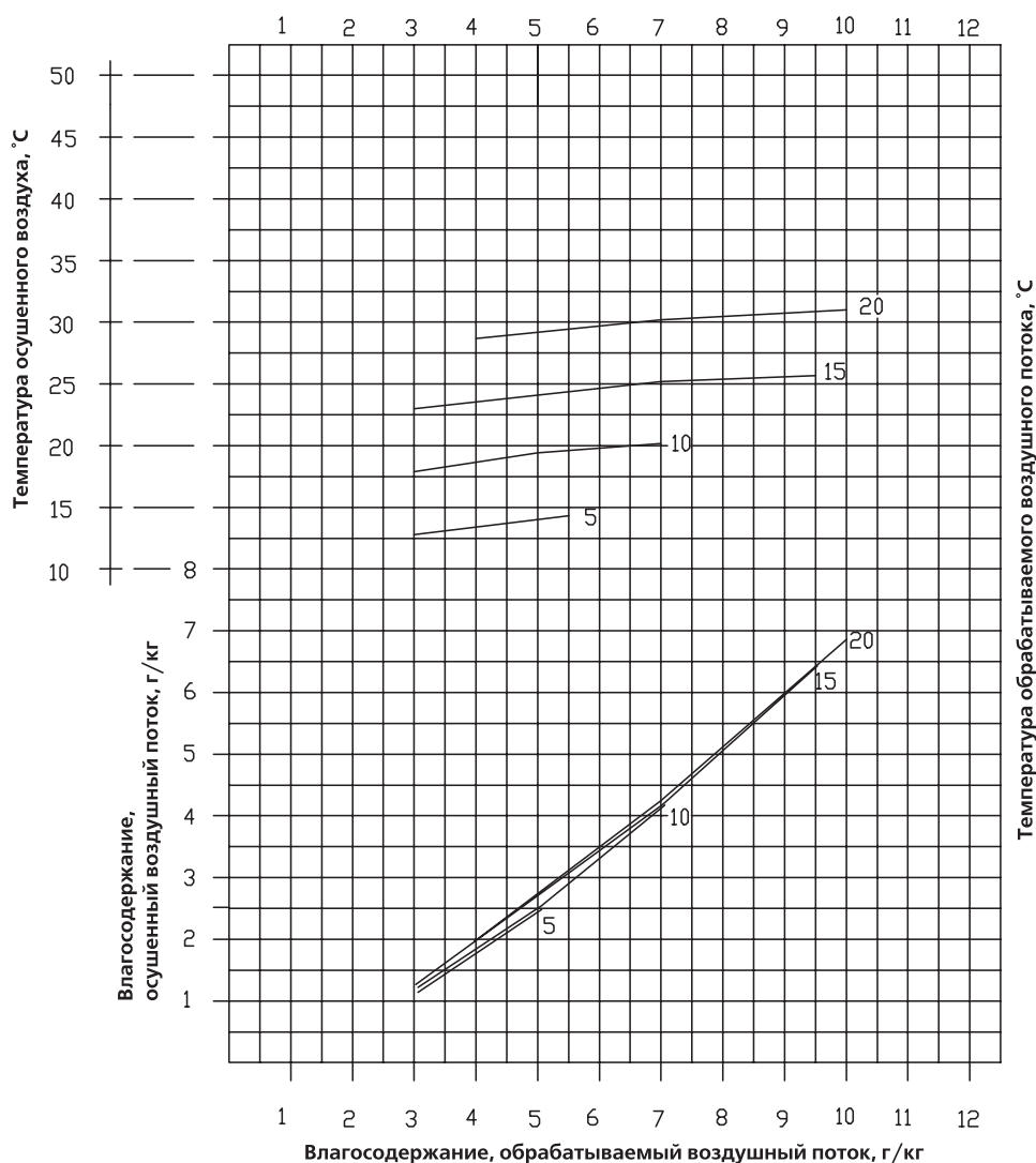
Номограмма 4: кривые влагосъема для осушителей CR240B/VT, CR300B/VT, 400B/VT
