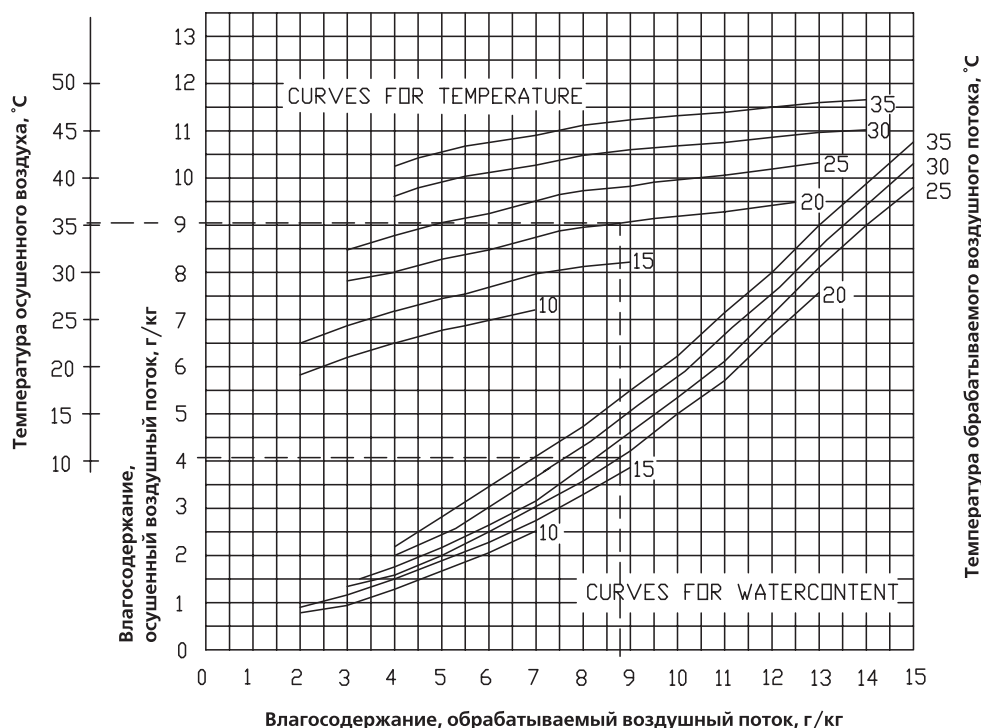
Номограмма 3: кривые влагосъема для осушителей CR80B, CR110B/VT, CR110LK, CR150B/VT, CR200B/VT
