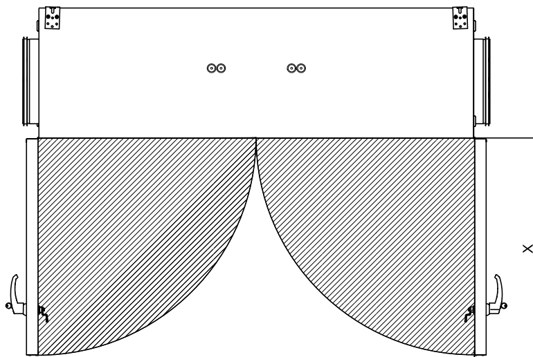
Рис. 2 Требуемое пространство
